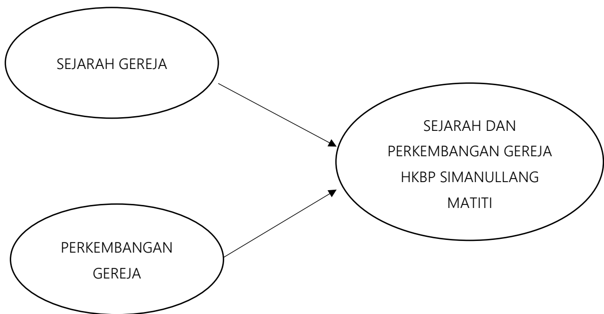
Gambar 1 kerangka konseptual
