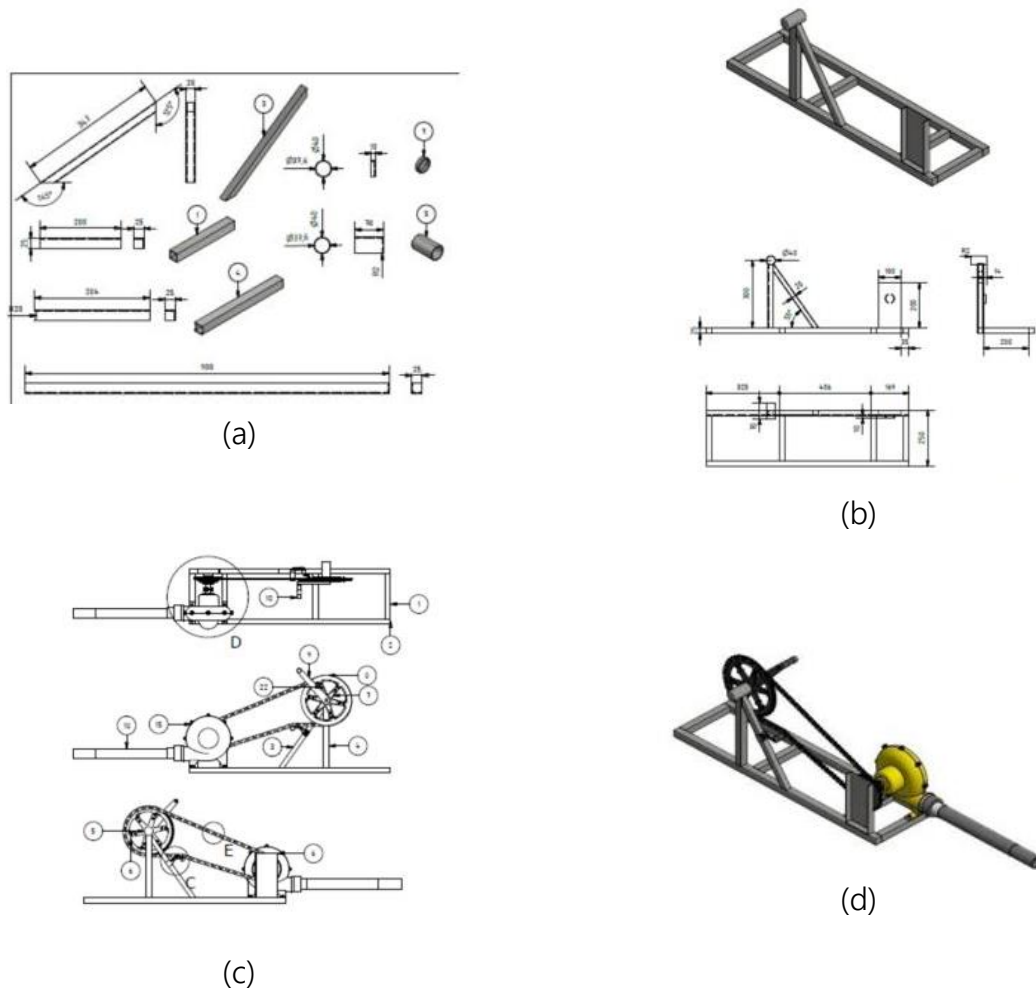
Gambar 2. Perancangan Alat Blower; (a) Perancangan Kerangka dan dudukan; (b) Perancangan Rangka; (c) Assembly rangka, blower manual, gear, rantai, cerobong, stabilizer dan baling baling; (d) Hasil assembly rangka dan blower.
