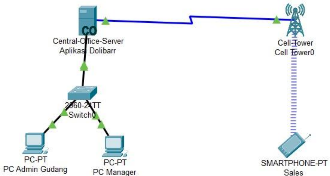
Gambar 6. Topologi Jaringan pada perusahaan Drinkdong
