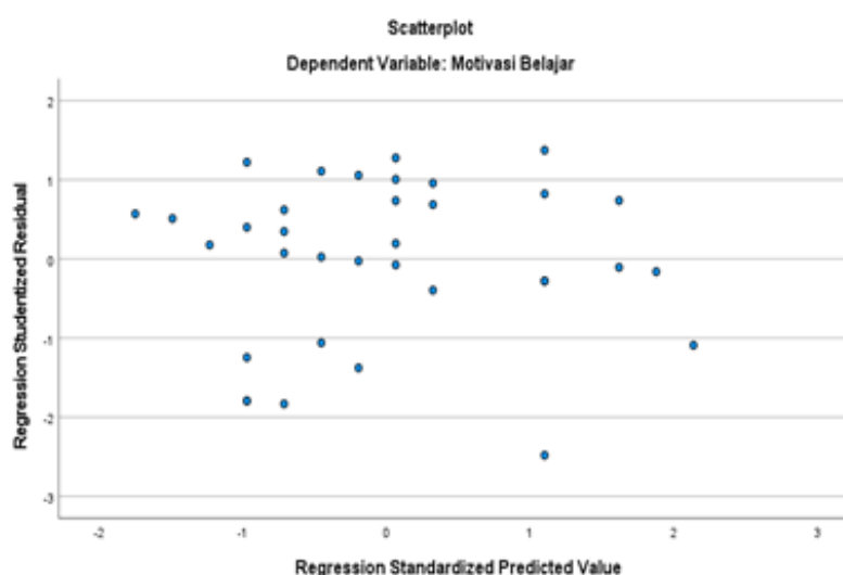
Gambar 2. Grafik Scatterplot
