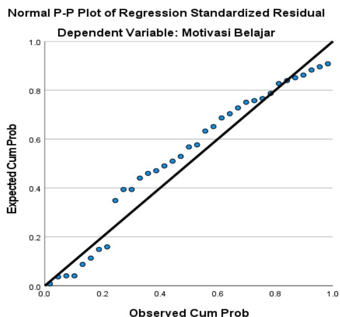
Gambar 1. P-plot
