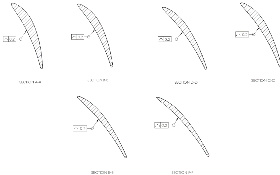
Gambar 2: Penerapan toleransi profil garis setiap section
