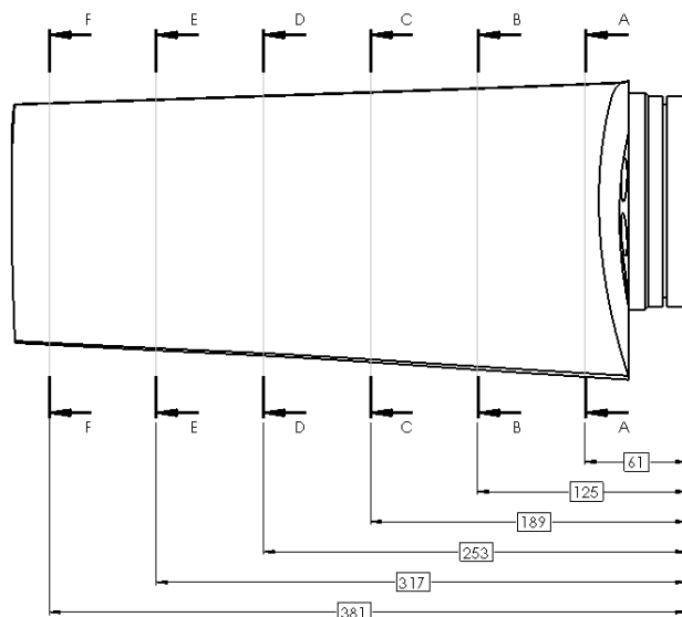
Gambar 1: Lokasi section penerapan toleransi profil garis
