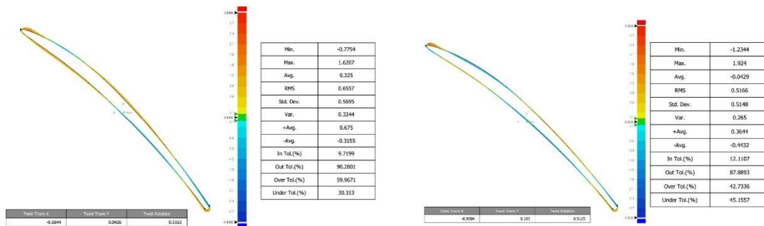
Gambar 4. Hasil inspeksi penyimpangan profil garis section C-C dan D-D
