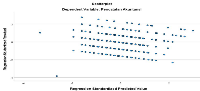
Gambar 2. Hasil Uji Heterokedasitas Grafik Scatterplot
