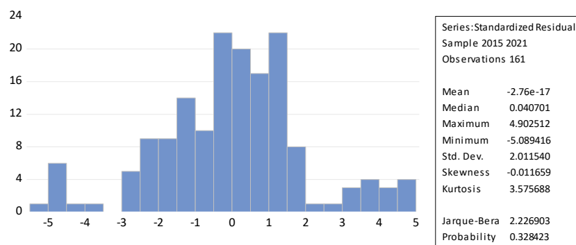
Gambar 2. Histogram Normalitas
