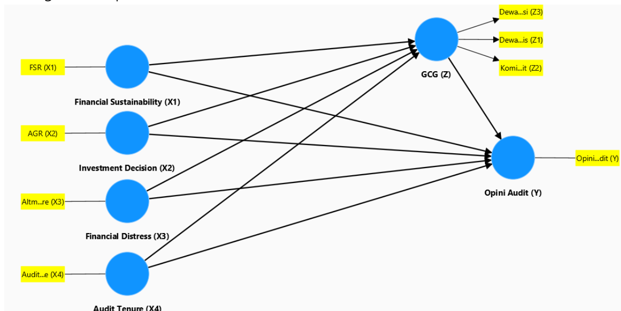
Gambar 1. Kerangka Konseptual
