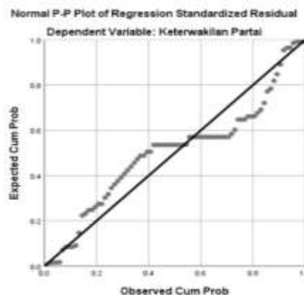
Gambar 1. Grafik P-P Plot Uji Normalitas
