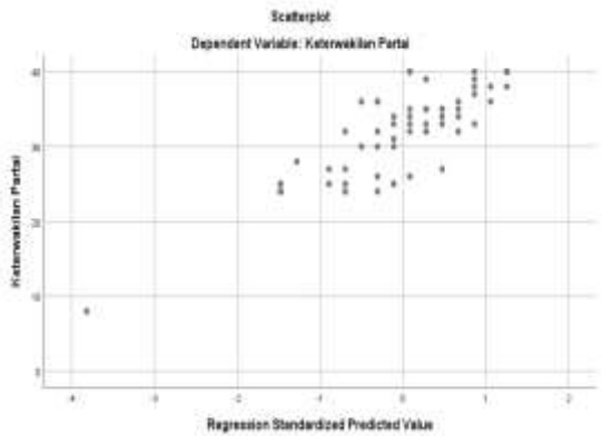
Gambar 2. Graffik Scatter Uji Heterokedastitas
