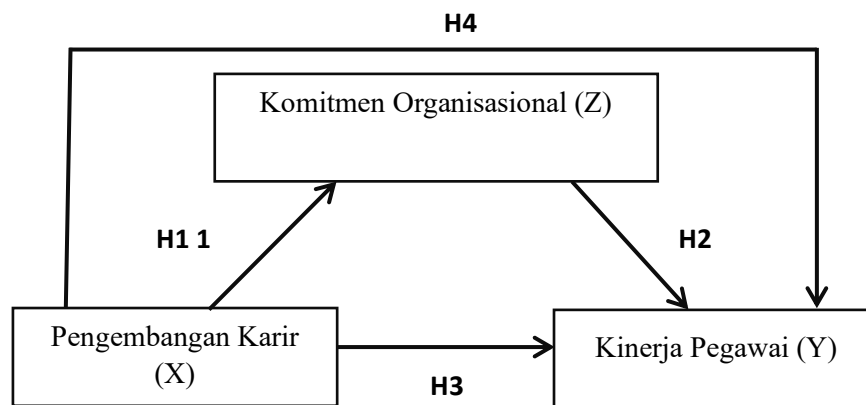
Gambar 1.1 Kerangka Konseptual
